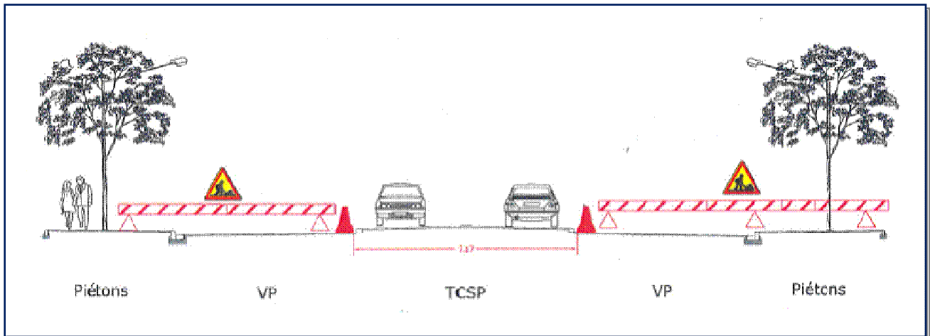
Coupe de la rue Camboulives entre le giratoire Basso-Cambo et le giratoire Marcel Achard
